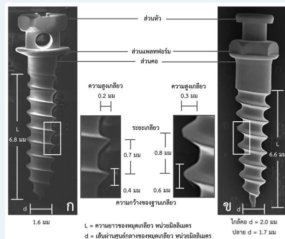
รูปที่ 1 หมุดเกลียวขนาดเล็กภาพจากกล้องจุลทรรศน์อิเล็กตรอนชนิดส่องกราดที่กำลังขยาย 8 เท่า ก) หมุดเกลียวขนาดเล็กทางการค้า ข) หมุดเกลียวขนาดเล็กที่ผลิตขึ้นเอง
