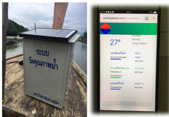
ภาพที่ 3 ระบบตรวจวัดคุณภาพน้ำต้นแบบและแอปพลิเคชันเพื่อการเฝ้าระวังคุณภาพน้ำและเตือนภัยบนโทรศัพท์มือถือ
