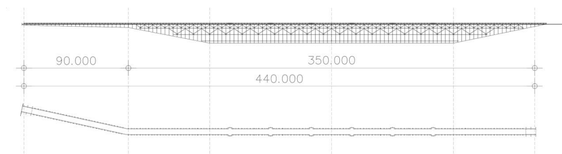
ภาพผังและรูปด้านของสะพานไม้อุตตมานุสรณ์
