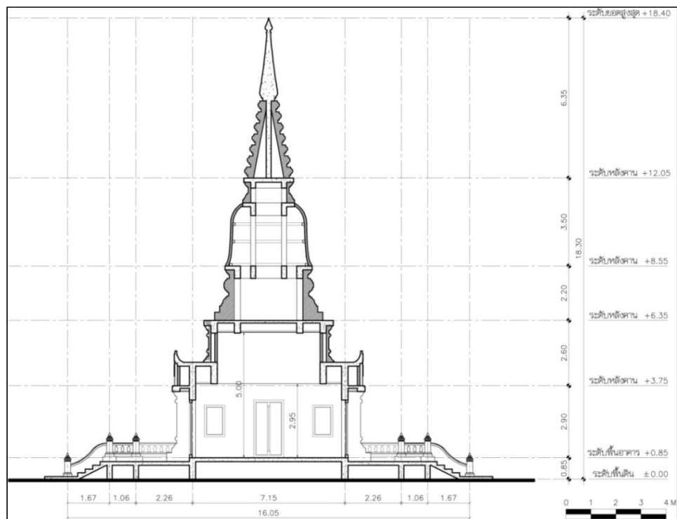
ภาพที่ 18 แบบสถาปัตยกรรม : รูปตัดพระเจดีย์
