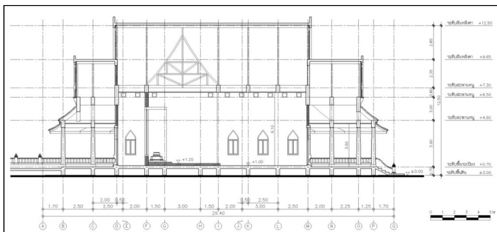
ภาพที่ 13 แบบสถาปัตยกรรม : รูปตัดพระอุโบสถ รูปตัด 1
