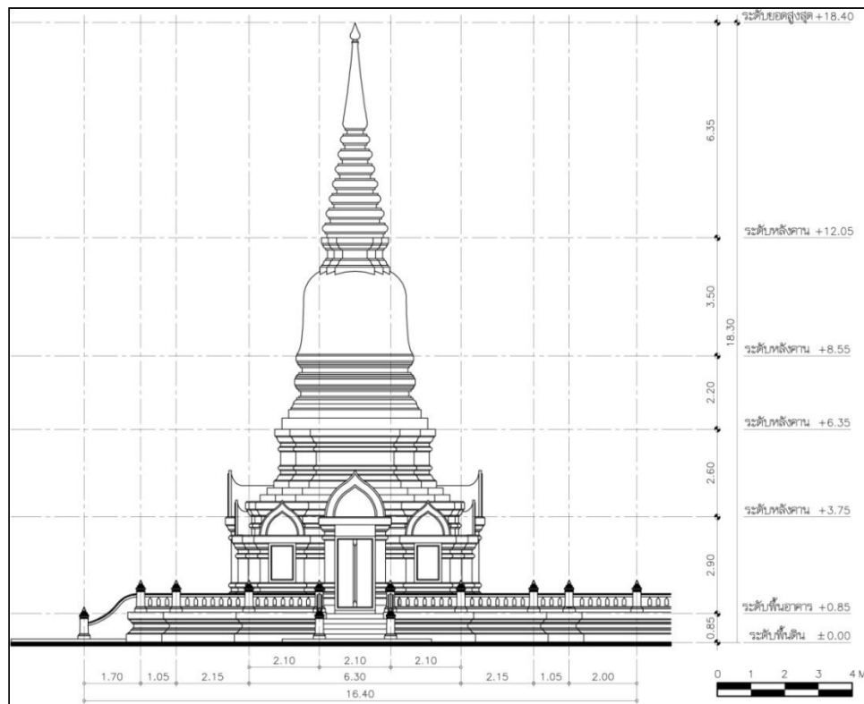
ภาพที่ 17 แบบสถาปัตยกรรม : รูปด้านพระเจดีย์
