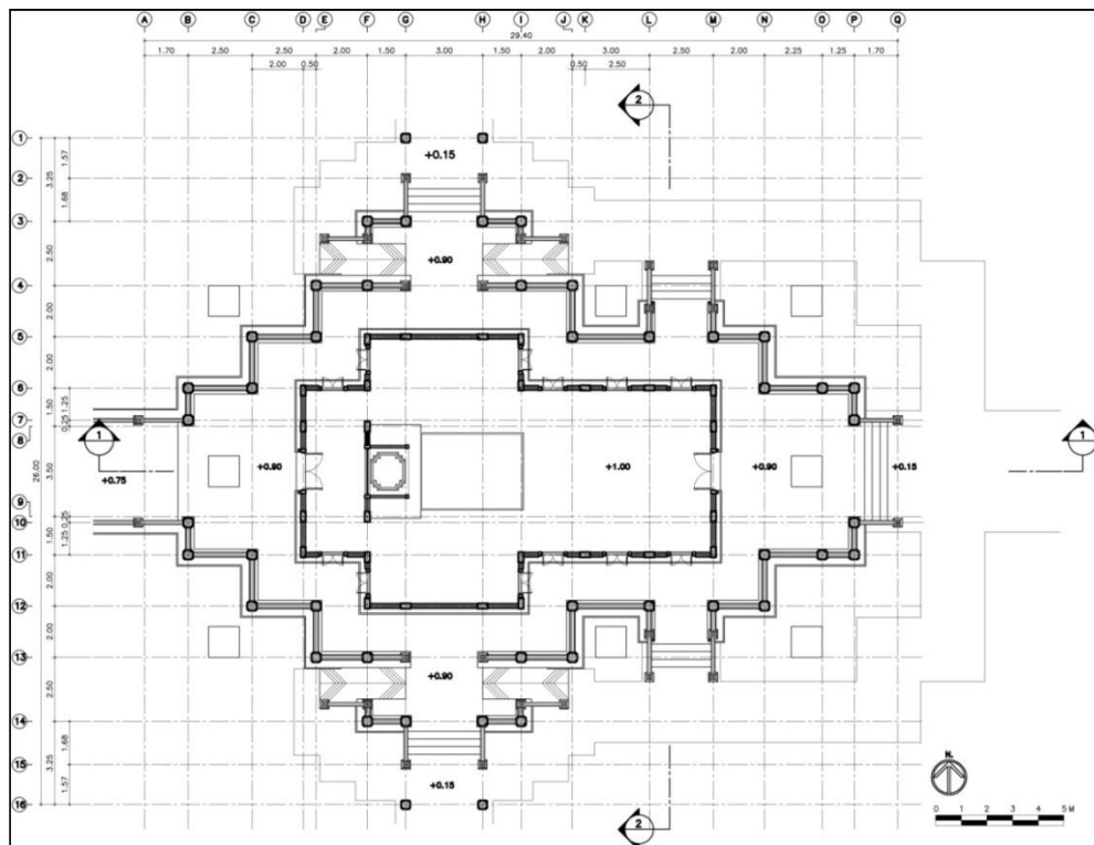
ภาพที่ 10 แบบสถาปัตยกรรม : ผังพื้นพระอุโบสถ
