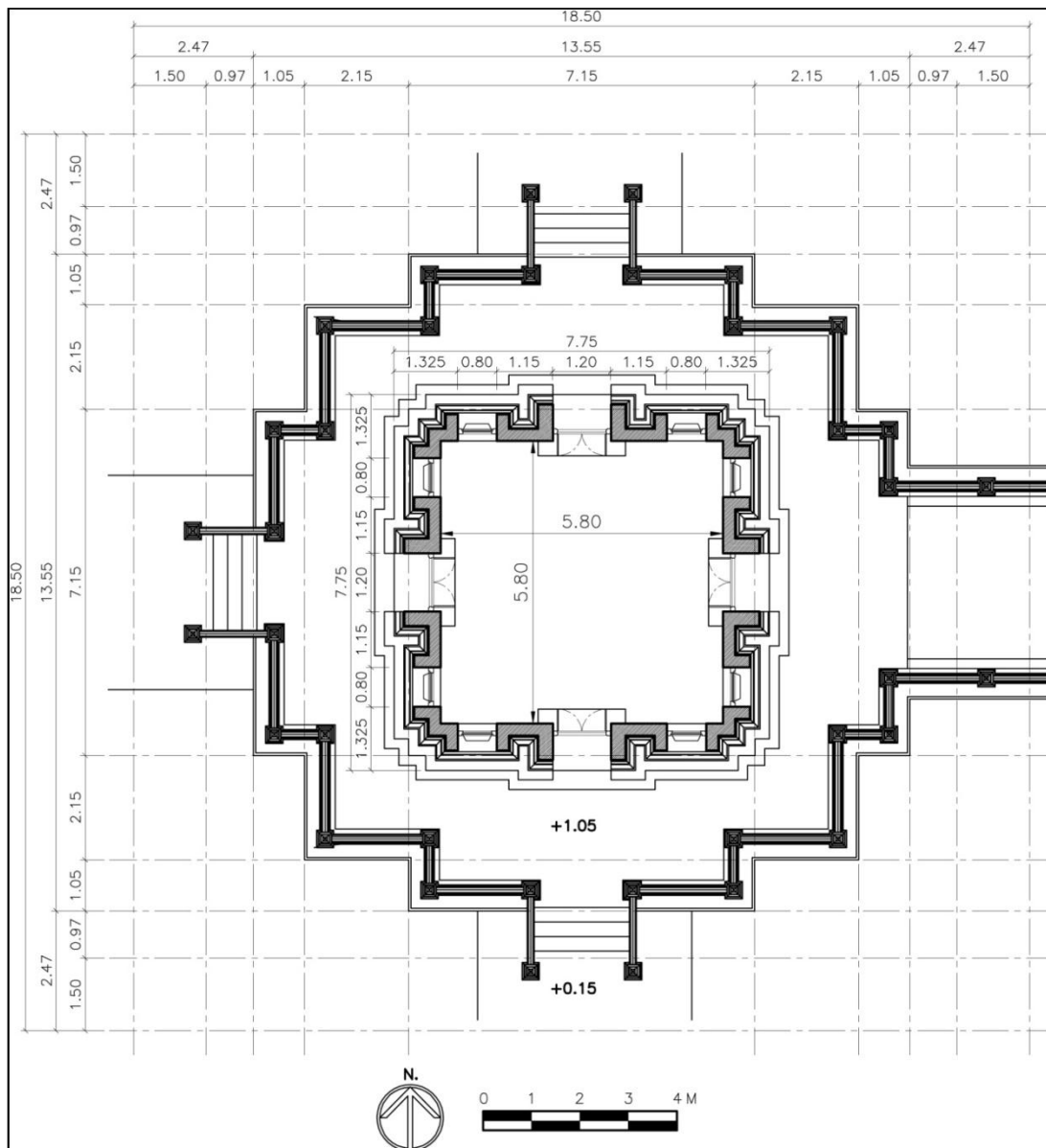
ภาพที่ 16 แบบสถาปัตยกรรม : ผังพื้นพระเจดีย์
