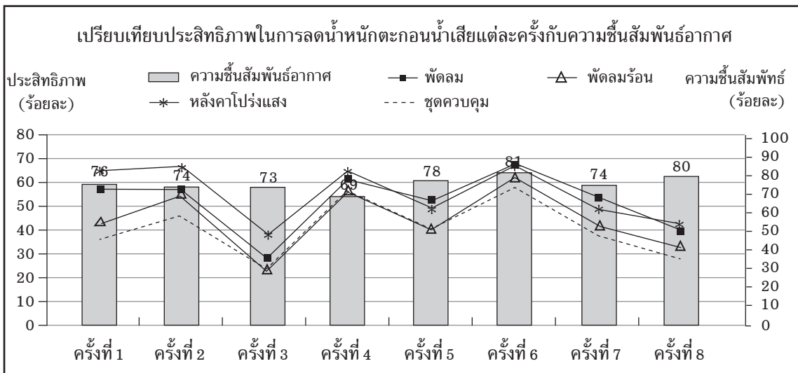
ภาพที่ 7 ประสิทธิภาพการลดน้ำหนักตะกอนน้ำเสียในแต่ละครั้งเปรียบเทียบกับความชื้นสัมพัทธ์อากาศ
