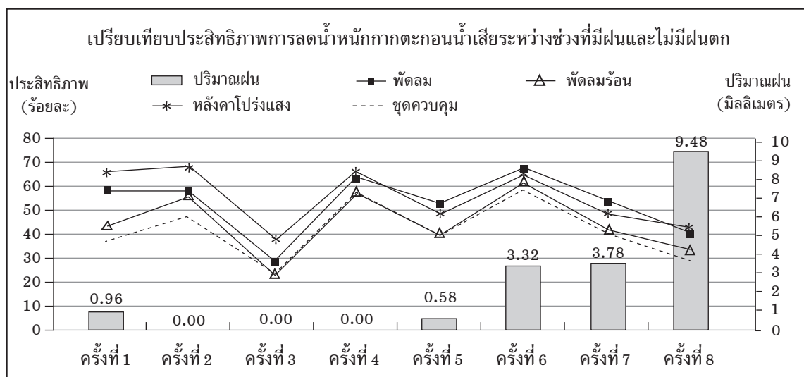
ภาพที่ 6 ประสิทธิภาพการลดน้ำหนักจากตะกอนน้ำเสียในแต่ละครั้งเปรียบเทียบระหว่างช่วงที่มีฝนและไม่มีฝน
