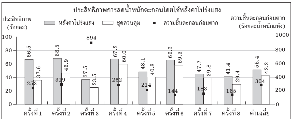
ภาพที่ 4 ประสิทธิภาพการลดน้ำหนักตะกอนน้ำเสียโดยใช้หลังคาโปร่งแสงเทียบกับความชื้นตะกอนก่อนการทดลอง
