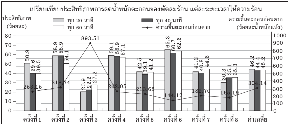
ภาพที่ 3 ประสิทธิภาพการลดน้ำหนักตะกอนน้ำเสียโดยใช้พัดลมร้อน ที่ระยะเวลาในการให้ความร้อนที่แตกต่างกันของการทดลองทั้ง 8 ครั้ง
