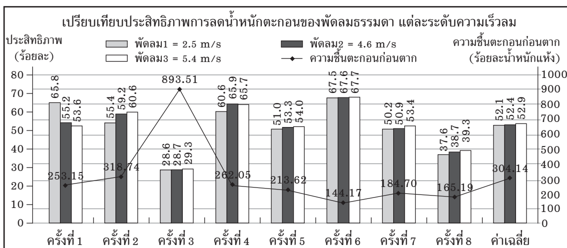
ภาพที่ 2 ประสิทธิภาพการลดน้ำหนักตะกอนน้ำเสียโดยใช้พัดลมธรรมดา ที่ระดับความเร็วของพัดลมที่ต่างกันของการทดลอง 8 ครั้ง
