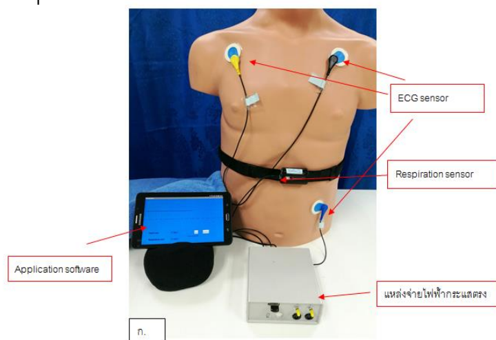
รูปที่ 7 แสดงลักษณะของเครื่องต้นแบบวัดการเต้นหัวใจและอัตราการหายใจ
